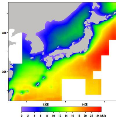
日本近海における波浪パワーの分布 (1994～2004年平均)
